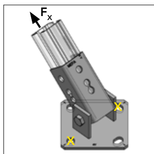
Scharnierconsole met voetplaat haaks Anker plaatsen bij X noodzakelijk
