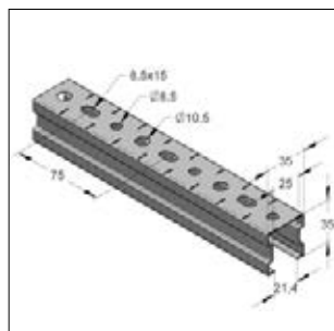
Montagerail 35/35
