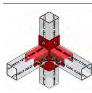
T-plaat
