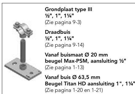
Onderdelen vastpunt
