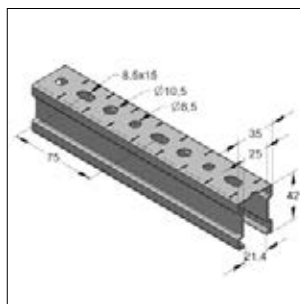
Montagerail 35/42
