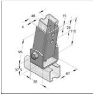
Scharnierhouder
