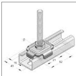
Combi profielhouder
