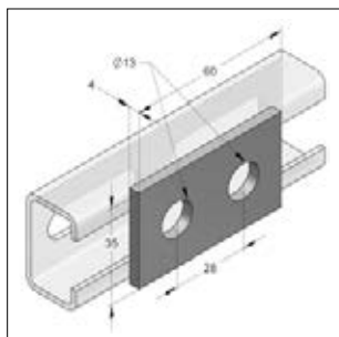
2-Gats verbindingsplaat 35/4
