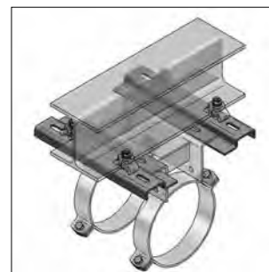
Montagevoorbeeld geleiderail 380
