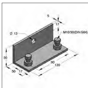
Draagklem
