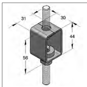
Hoogteversteller
