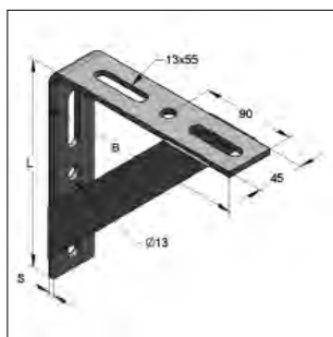
Hoekconsole
