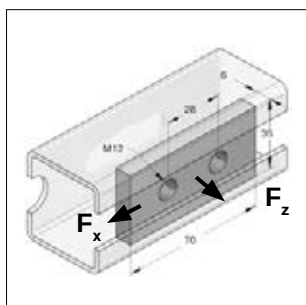
Montagemoer 2-gats
