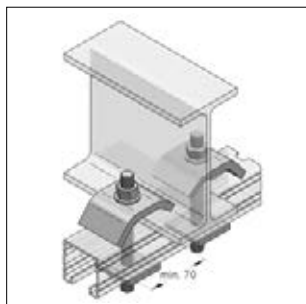
Spanklauw montageset
