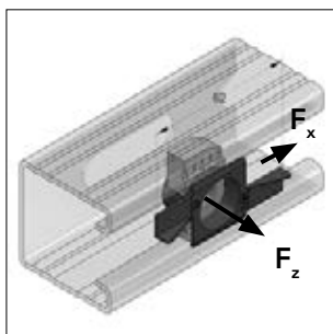
Stex 45 schuifmoer MP-X
