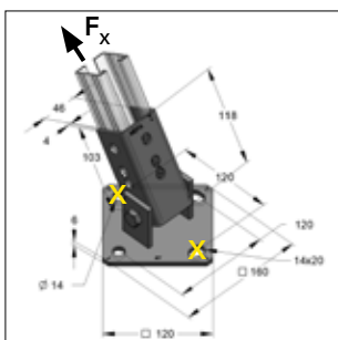
Scharnierconsole met voetplaat recht Anker plaatsen bij X noodzakelijk
