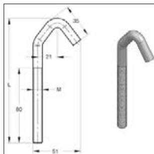
Draadhaak
