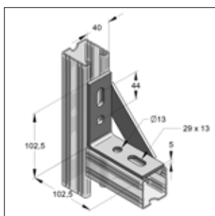
Hoekverbinder
