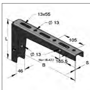
Universeel console
