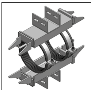
Vastpunt type B met CENTUM® stabiele lasuitvoering
