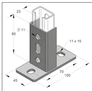
Houder 35 recht voor montagerail
