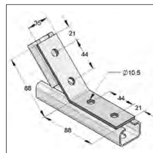
Hoekstuk 35/4 4-gats 135°
