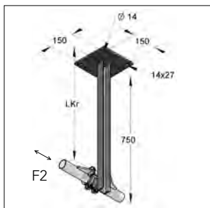
Vastpuntconsole 50/38/750
