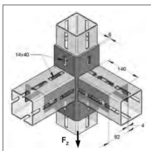
CENTUM® Hoekverbinder 90°
