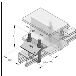
balkklemset M10 45/45
