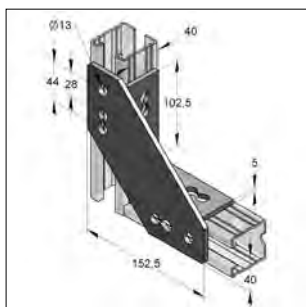
Universele hoekverbinder
