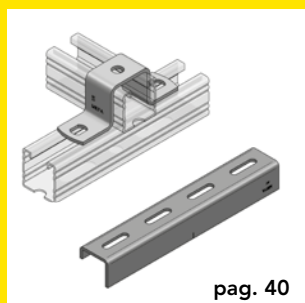
Klemverbinder Verbindingsstuk 45
