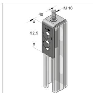
Eindhoeak aansluitstuk rail 45/45
