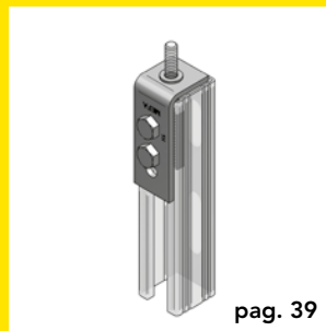
Eindhoek aansluitstuk 45/45
