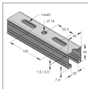
Montagerail C-profiel 45/45
