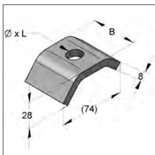
Spanklauw
