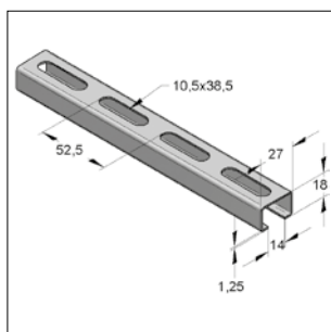
Montagerail C-profiel 27/18
