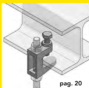
Balkklem C-model
