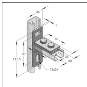
Montage(eind)plaat 35/4 recht
