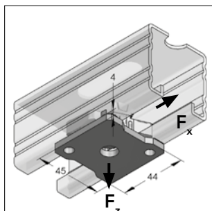
Stex 45 Schuifmoer
