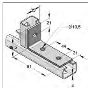
Hoekstuk 35/4 3-gats
