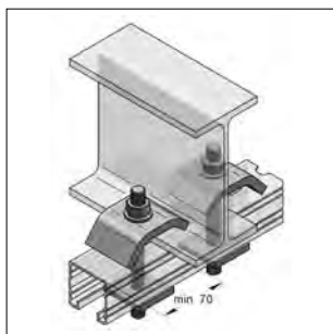
Spanklauw montageset
