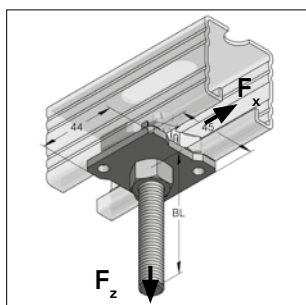
Stex 45 Hamerkopbout
