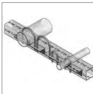
Montagevoorbeeld
