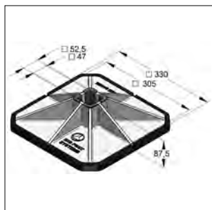
Daksteun BIG FOOT® 305 mm (inclusief EPDM onderlaag)
