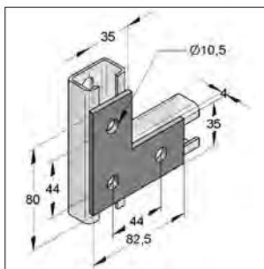
Verbindingsplaat 35/4 L-vorm
