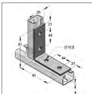
Hoekstuk 35/4 4-gats 90°
