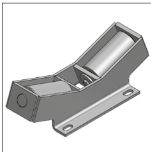
Roldrager dubbel axiaal
