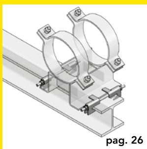
Geleidingklem-set
