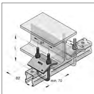
balkklemset M8 35
