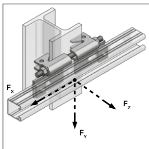
Balkklem verticaal
