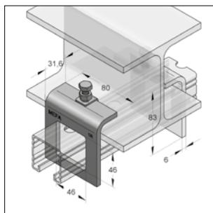
Balkklem
