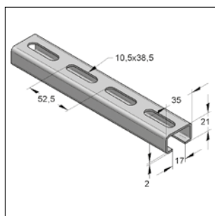
Montagerail C-profiel 35/21
