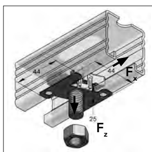
Stex 45 Montagebout
