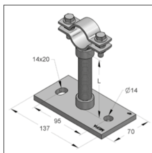
Klemvastpunt
