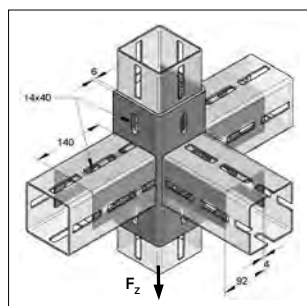
CENTUM® Hoekverbinder 180°
