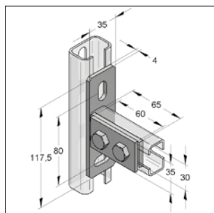
Montage(eind)plaat 35/4 haaks
