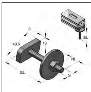
Hamerkopbout
