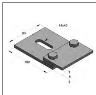
CENTUM® Z-houder Klumbereik 11 mm
