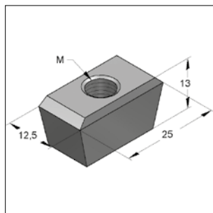
keilmoer voor profielplaat
