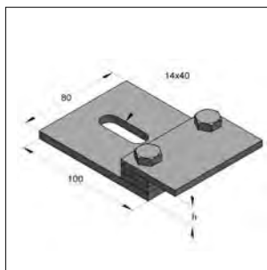
CENTUM® Z-houder Klumbereik 16 mm
