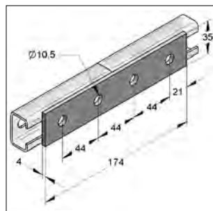
Verbindingsplaat 35/4 4-gats
