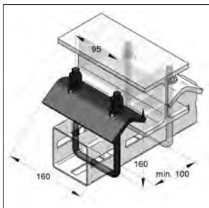
CENTUM® Balkklemset lichte uitvoering
