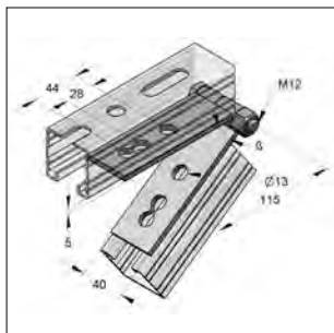
Scharnierverbinder
