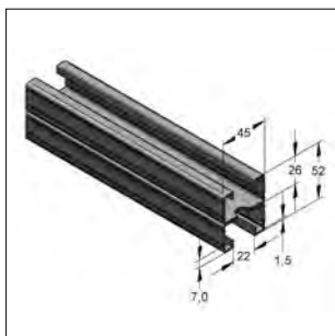
Montagerail C-profiel 45/52
