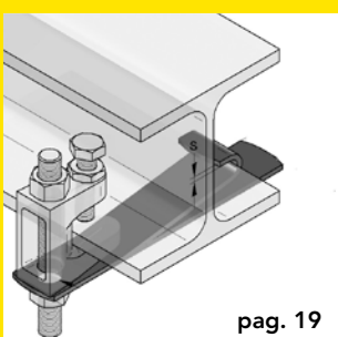
Veiligheidsstrip
