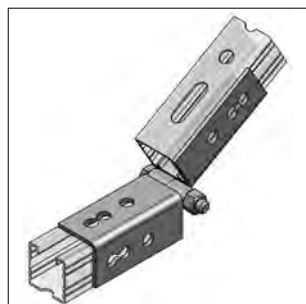
Profielhoek willekeurig
