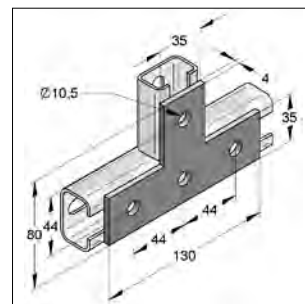
Verbindingsplaat 35/4 T-vorm
