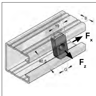
Montagemoer
