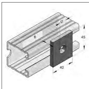
Verbindingsplaat
