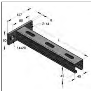
Console C-profiel 45/45/2,0 haaks
