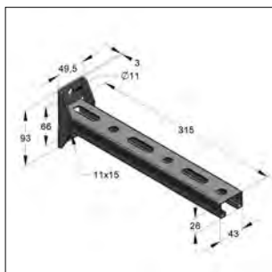
Console C-profiel 45/26/1,5 mm S
