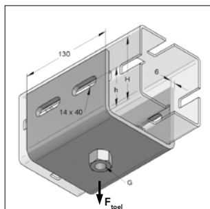
CENTUM® Profielloer aansluiting zwaar, XL 100 M16
