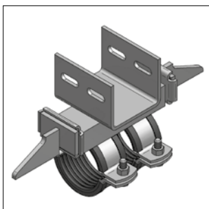
Vastpunt type A met CENTUM® stabiele lasuitvoering
